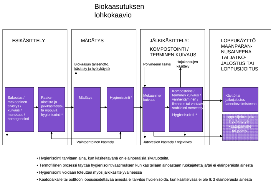
Kuva 2. Biokaasutusprosessi
